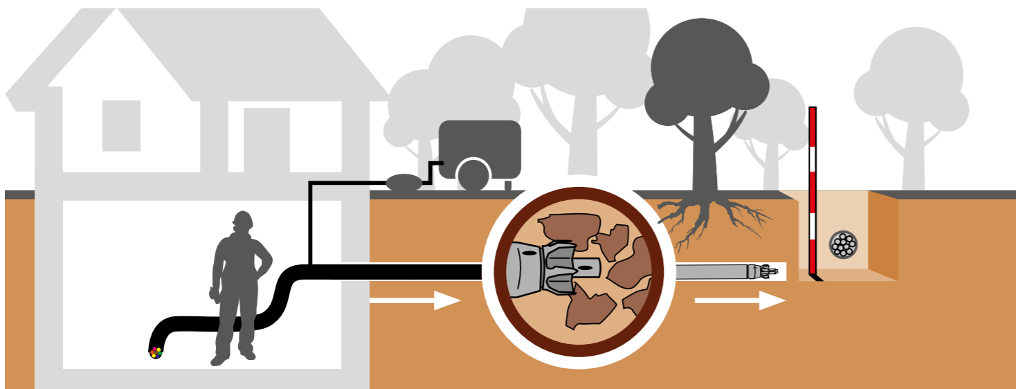
1. varianta NEŘÍZENÝ vrt do 15 m délky
